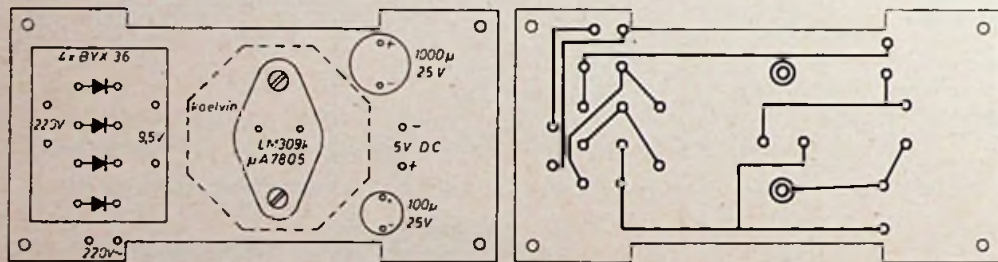
Boven: fig. 1. Hiernaast: fig. 4a en b, het printje is op halve grootte afgebeeld. Links onder: fig. 2. Rechts onder: fig. 3
